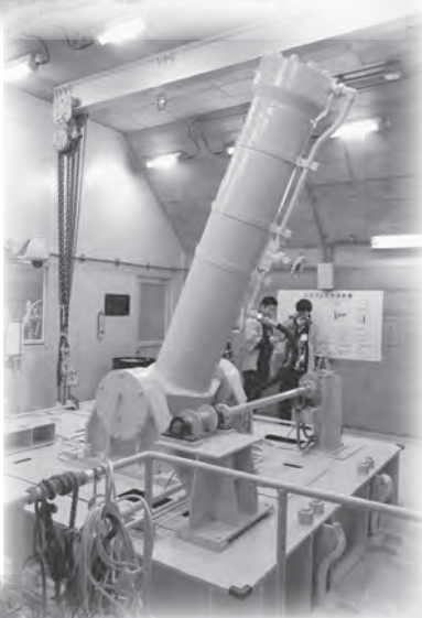
▶ダムの主ゲートを操る開閉装置
