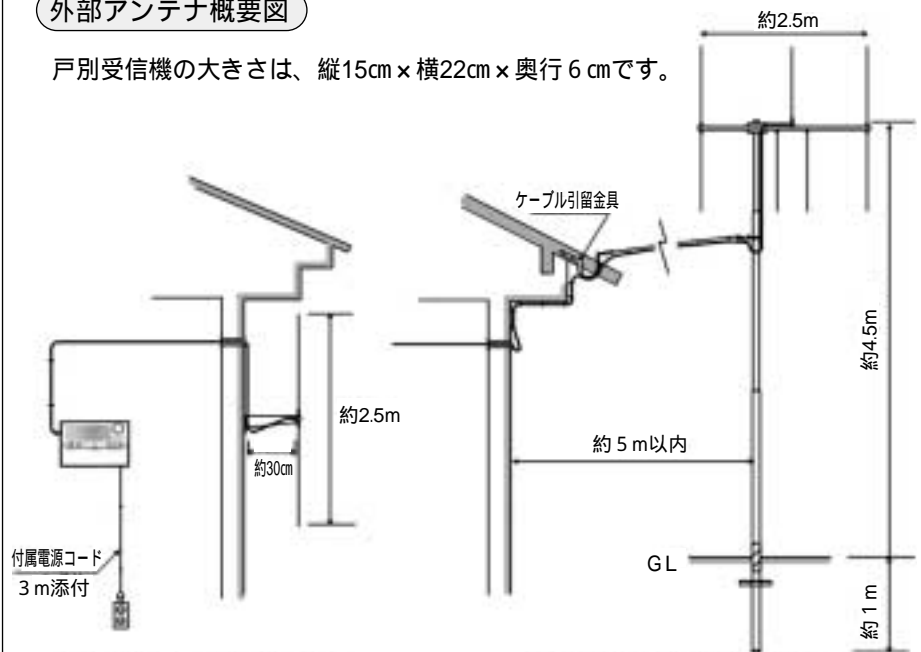
ダイポールアンテナ標準戸別受信機取付図
