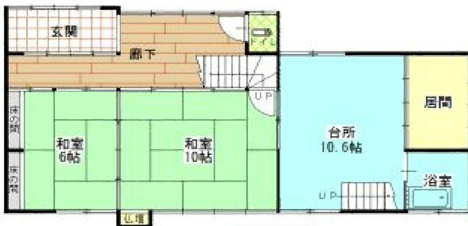
1階平面図
